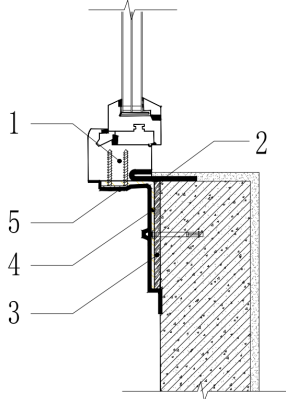
图 B.0.24 防水隔汽膜“U”字型粘贴示意图
