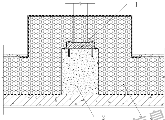
图 B.0.28 超低能耗居住建筑边界的屋面连接设备基础断热桥措施做法 2
