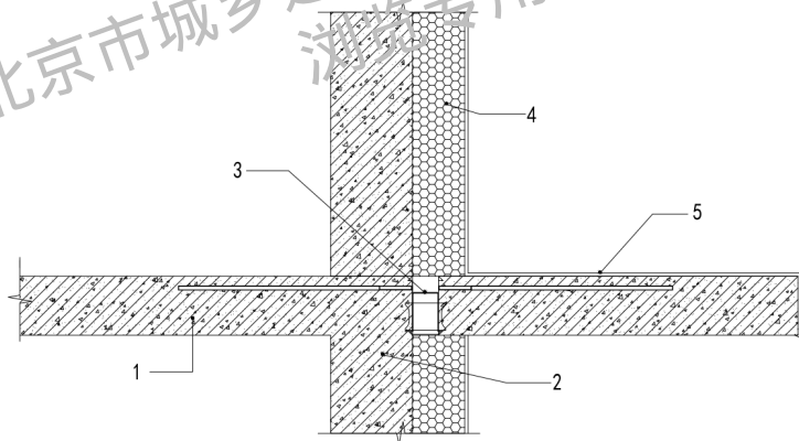
图 B.0.3 阳台板断热桥承重连接件做法
