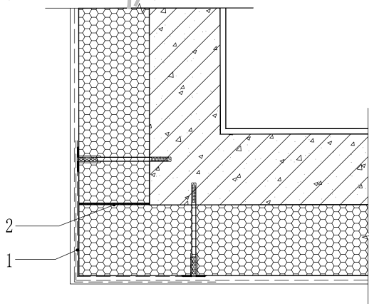
图 B.0.13 阳角处增强做法
