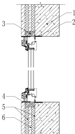
图 B.0.18 装配式建筑外窗安装
