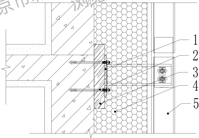
图 B.0.29 幕墙光伏系统断热桥做法
