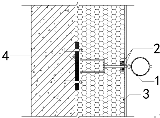
图 B.0.2 落水管处做法示意图
