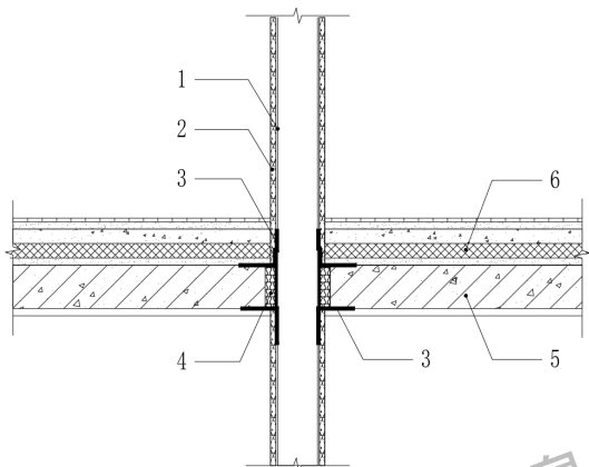
图 B.0.22 穿楼面管道断热桥做法
