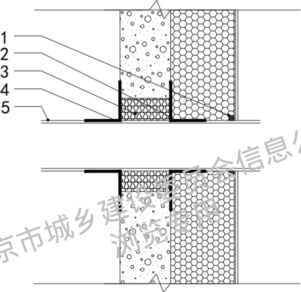
图 B.0.1 穿墙管处做法示意图
