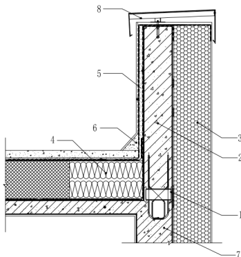
图 B.0.21 女儿墙断热桥承重连接件做法
