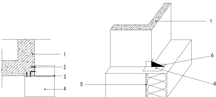
图 B.0.7 阳角托架安装
