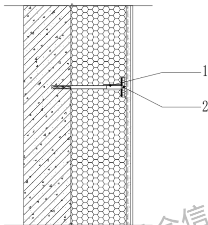
图 B.0.12 断热桥锚栓沉入式安装示意图
