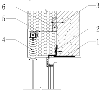
图 B.0.19 活动外遮阳安装示意图
