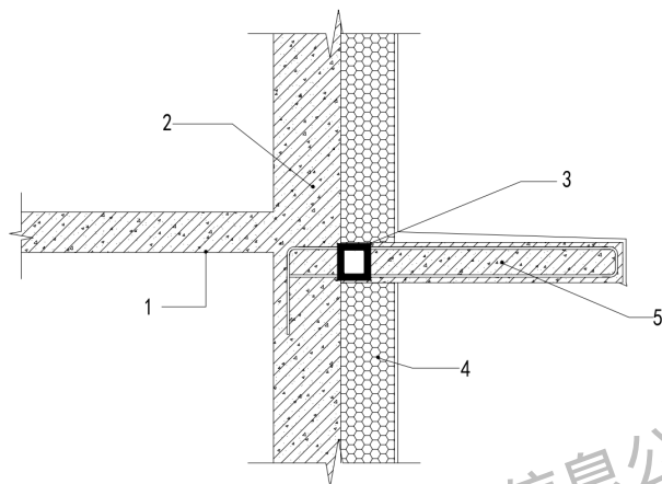
图 B.0.4 空调板断热桥承重连接件做法
