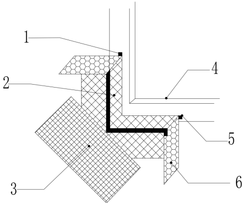
图 B.0.9 窗框外侧保温做法
