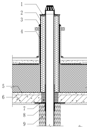
图 B.0.20 出屋面管道做法
