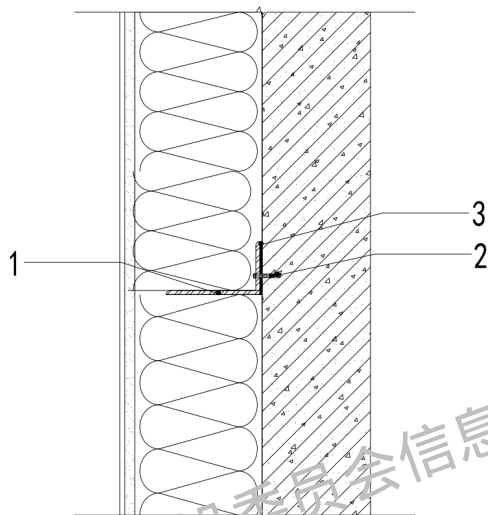
图 B.0.6 层间或起步托架安装
