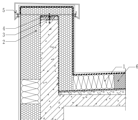
图 B.0.14 女儿墙保温及压顶板做法
