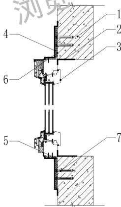
图 B.0.15 外窗外挂式安装-底部采用连接件固定
