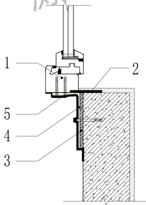
图 B.0.23 防水隔汽膜“一”字型粘贴示意图
