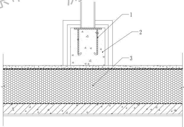
图 B.0.27 超低能耗居住建筑边界的屋面连接设备基础断热桥措施做法 1
