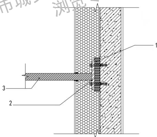
B.0.5 空调支架做法示意图
