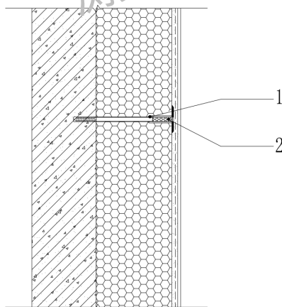
图 B.0.11 断热桥锚栓非沉入式安装示意图
