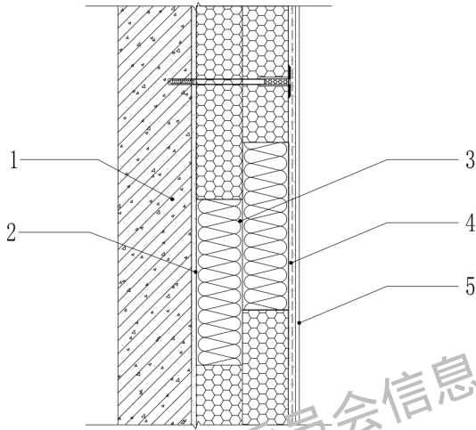
图 B.0.8 防火隔离带分层铺贴
