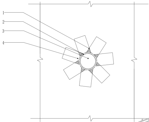
图 B.0.26 管道部位防水隔汽膜粘贴图
