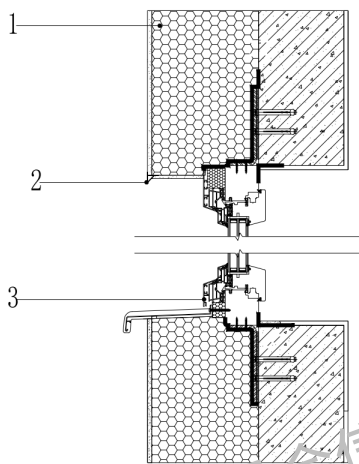
图 B.0.10 窗洞口保温做法剖面图
